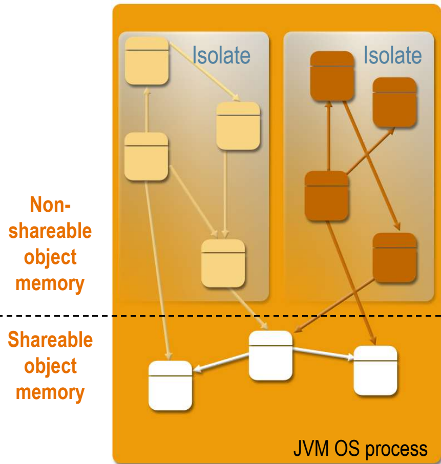
Squawk Java VM
